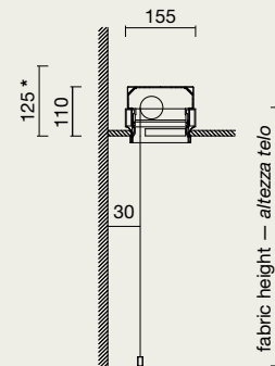
Fabric lowering: behind Discesa telo: dietro
